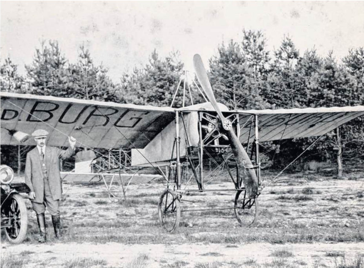
Hein van der Burg bij zijn toestel dat lichtjes gebaseerd op de Franse Blériot. Het had een houten, niet verstelbare propeller. De propeller zat vast aan de rotatiemotor. De gehele motor, inclusief de propeller, draaide in de rondte. De krukas zat aan het vliegtuig vast. De staart is de nationale driekleur geschilderd.
